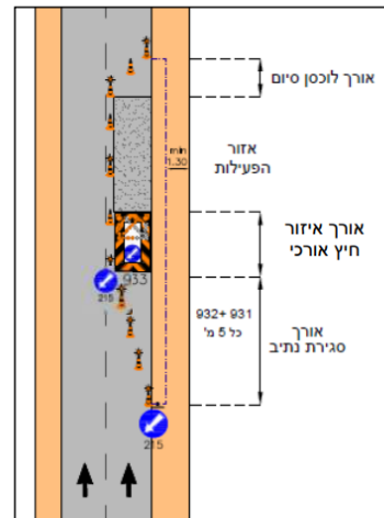
איור 2.3.13: סגירת נתיב ימין באמצעות לוכסן
